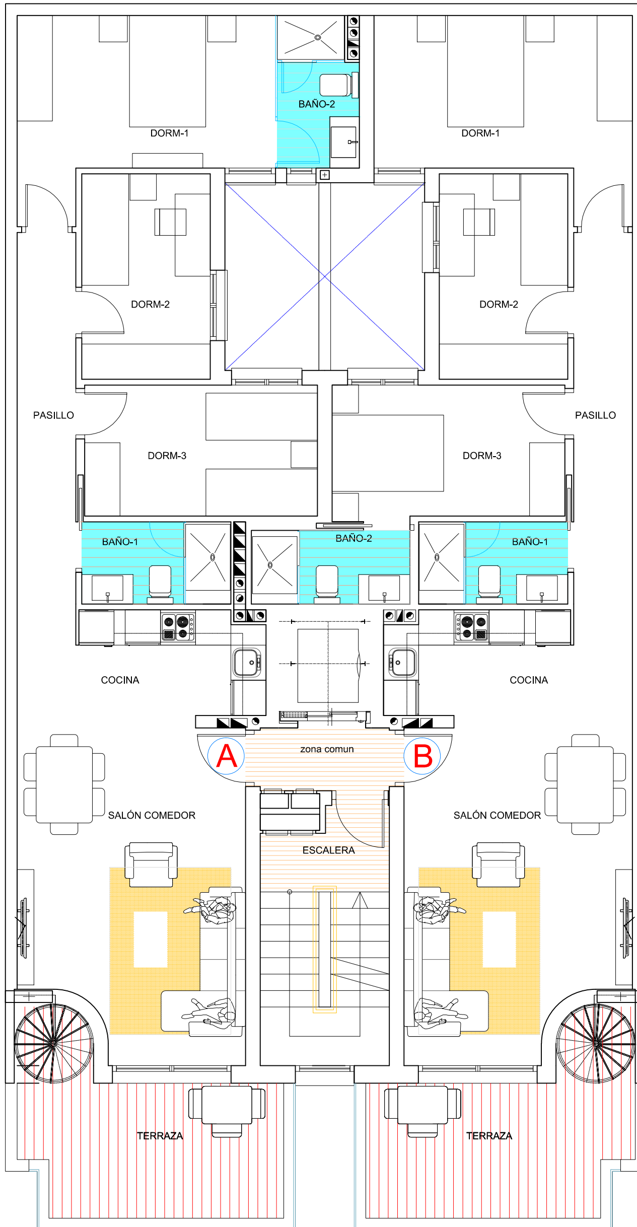
PLANTA ATICO
