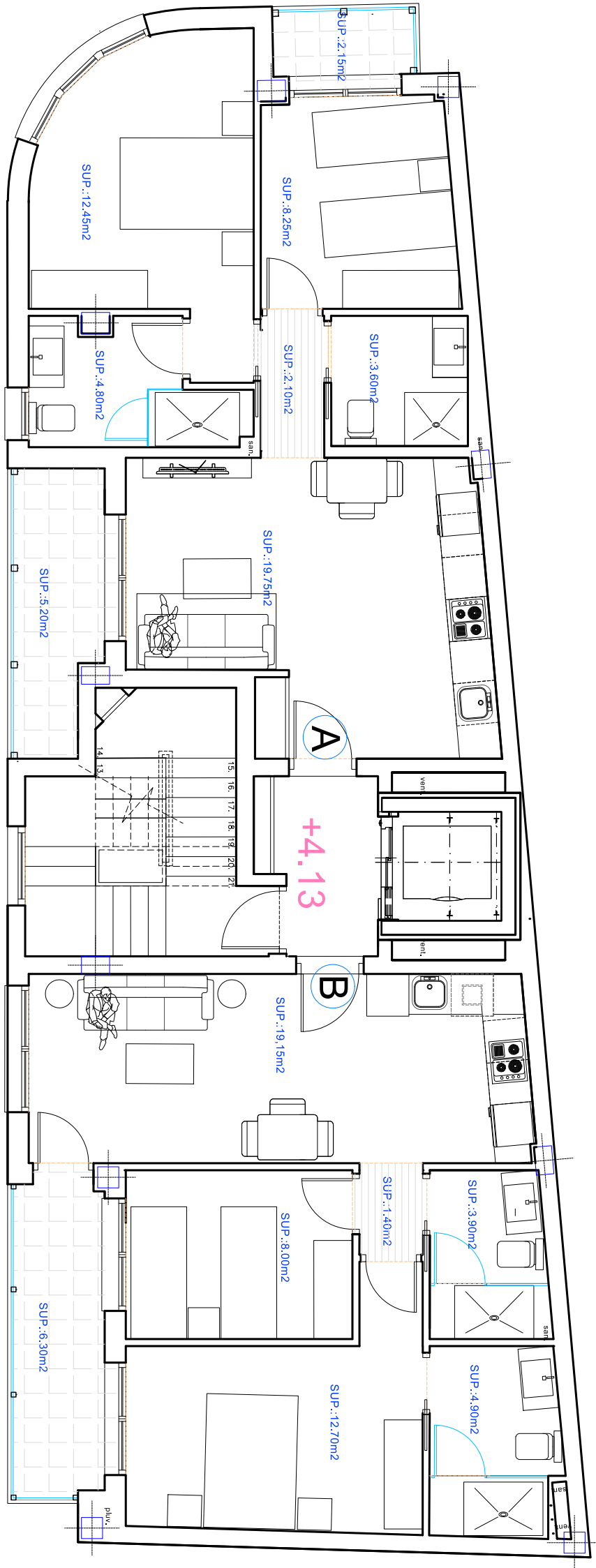
PLANTA PRIMERA
