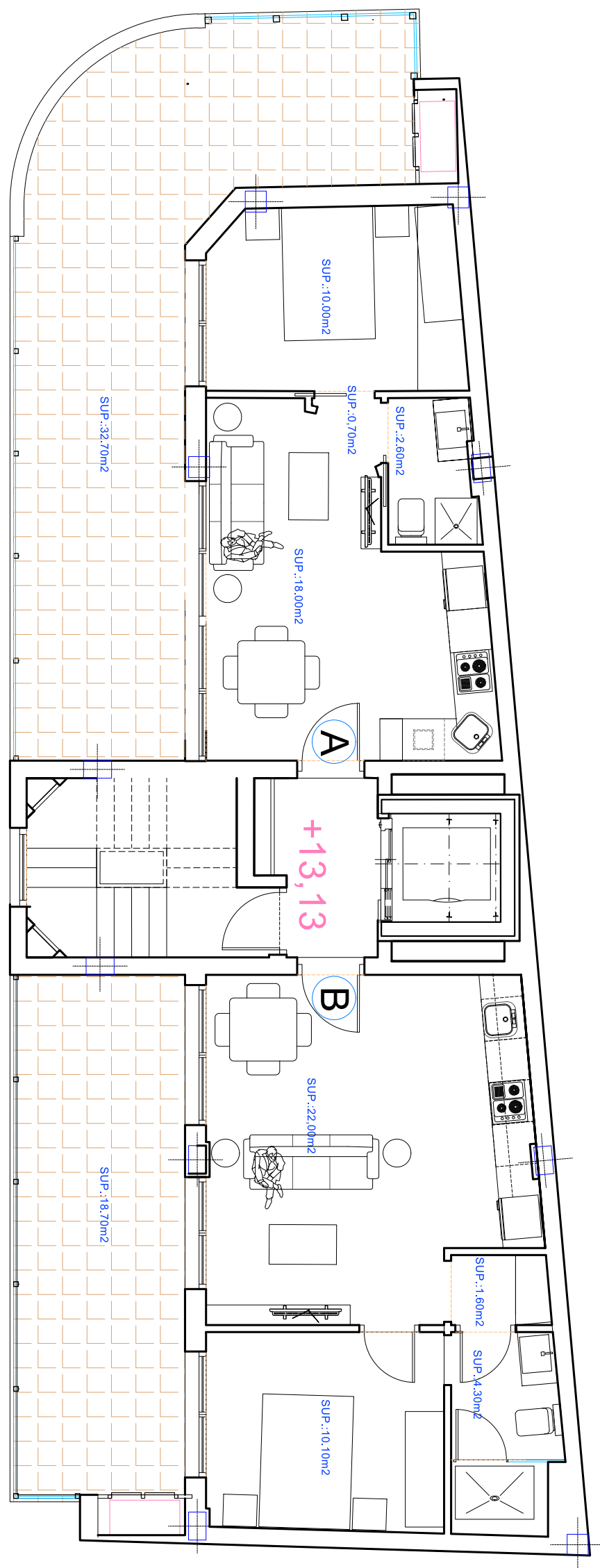
PLANTA ATICO
