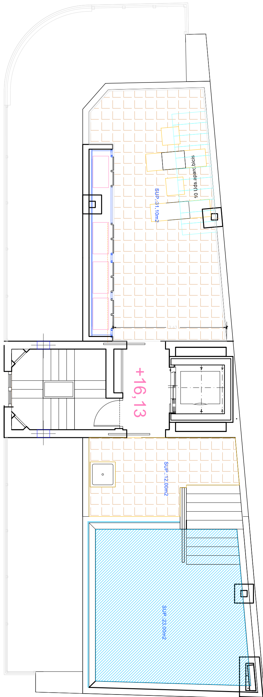
PLANTA CUBIERTA
