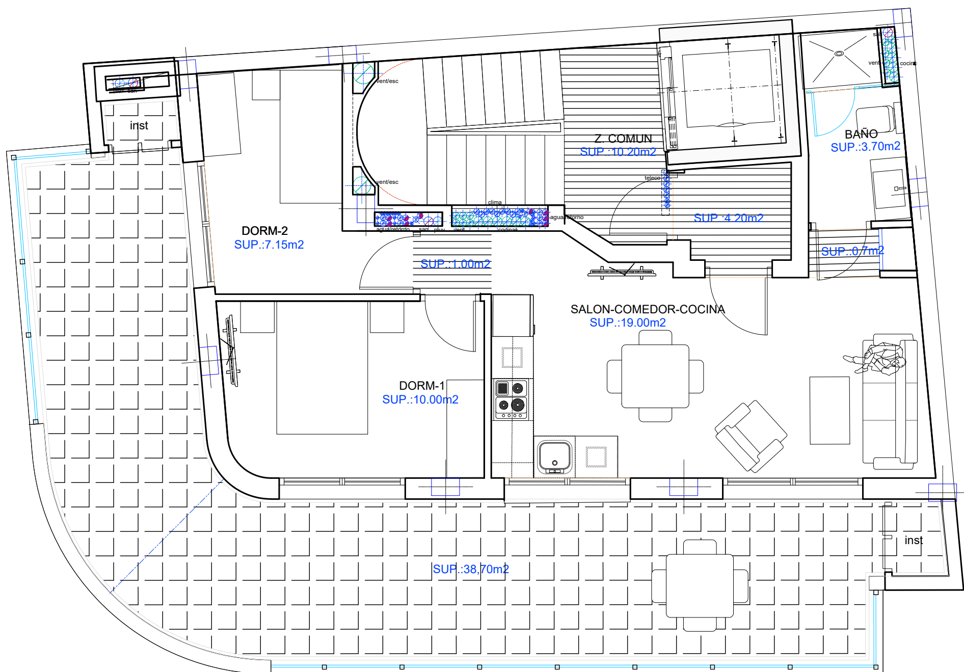
PLANTA ATICO
