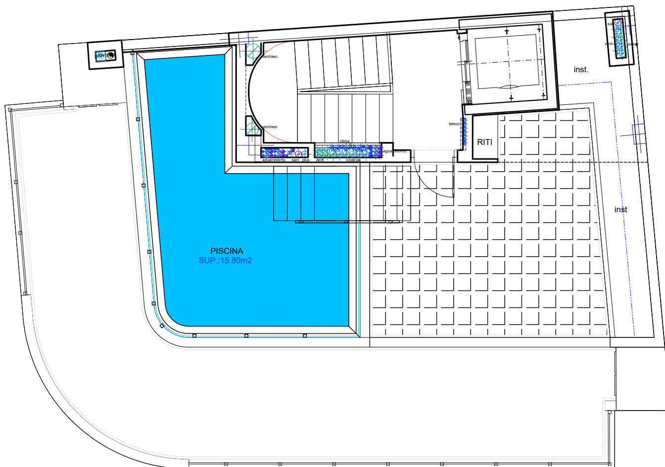
PLANTA CUBIERTA
