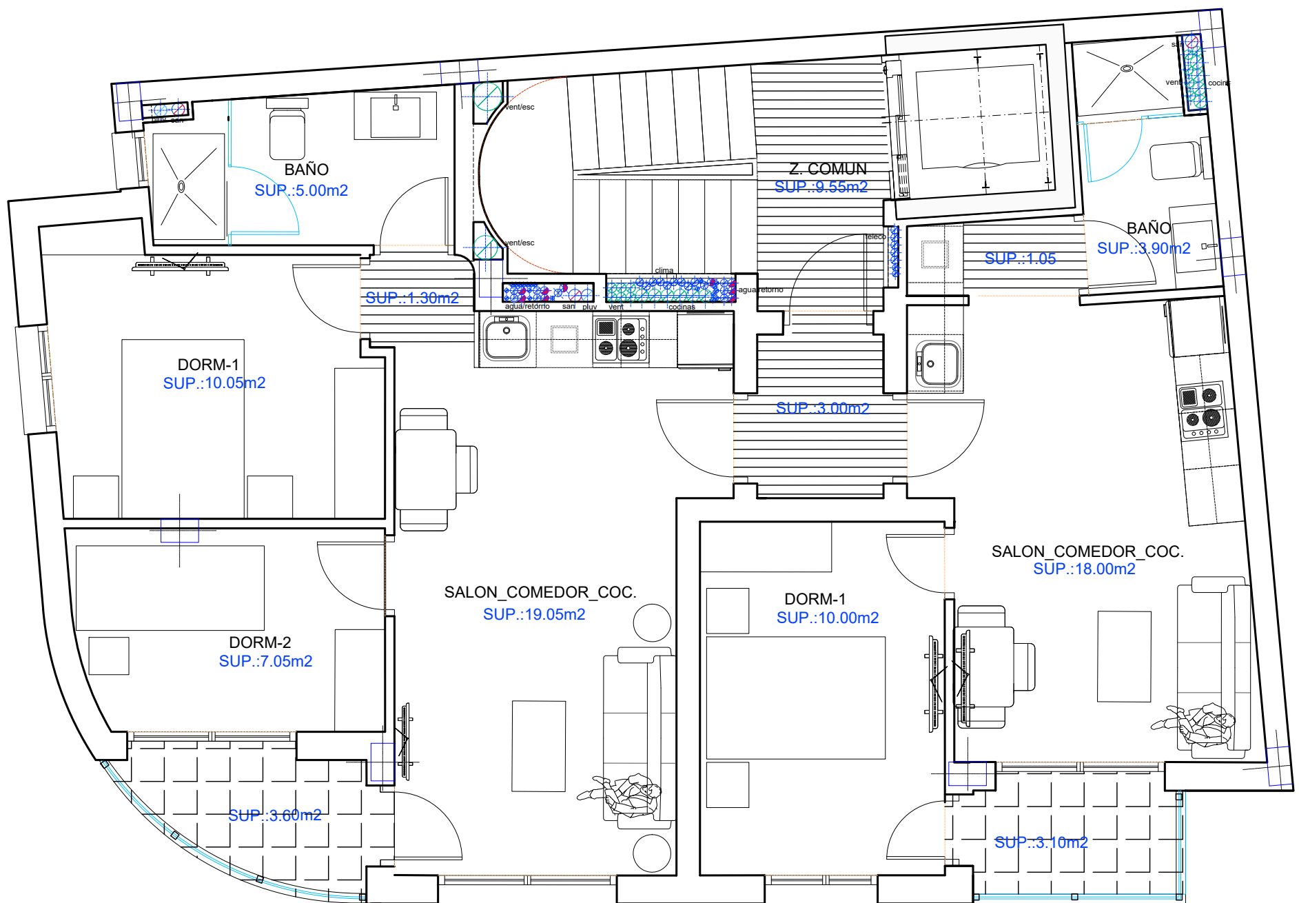
PLANTA 1-4
